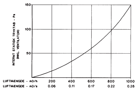
IF-OILMASTER TYPE 1000 TOTALT TRYKTAB VED RENE FILTRE
